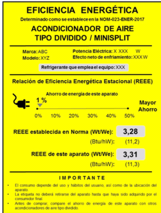
Figura A.9 - Ejemplo de etiqueta para acondicionadores de aire descarga libre sin conductos
