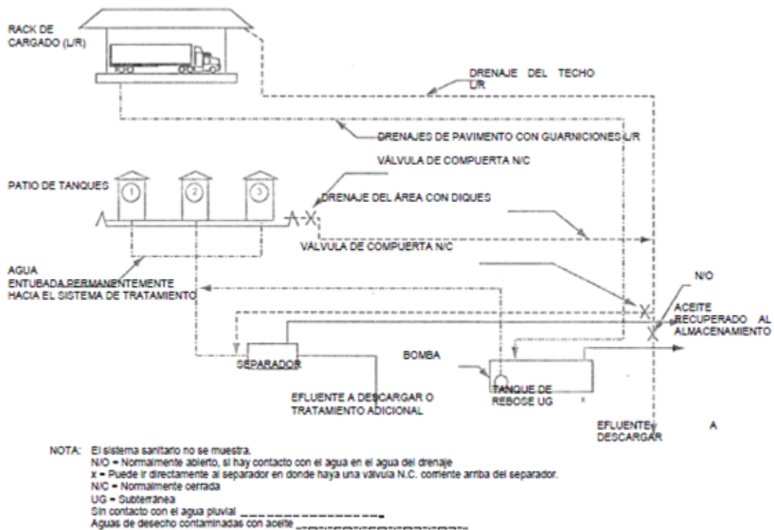
Figura 10. Sistema de Drenaje pluvial y aceitoso
