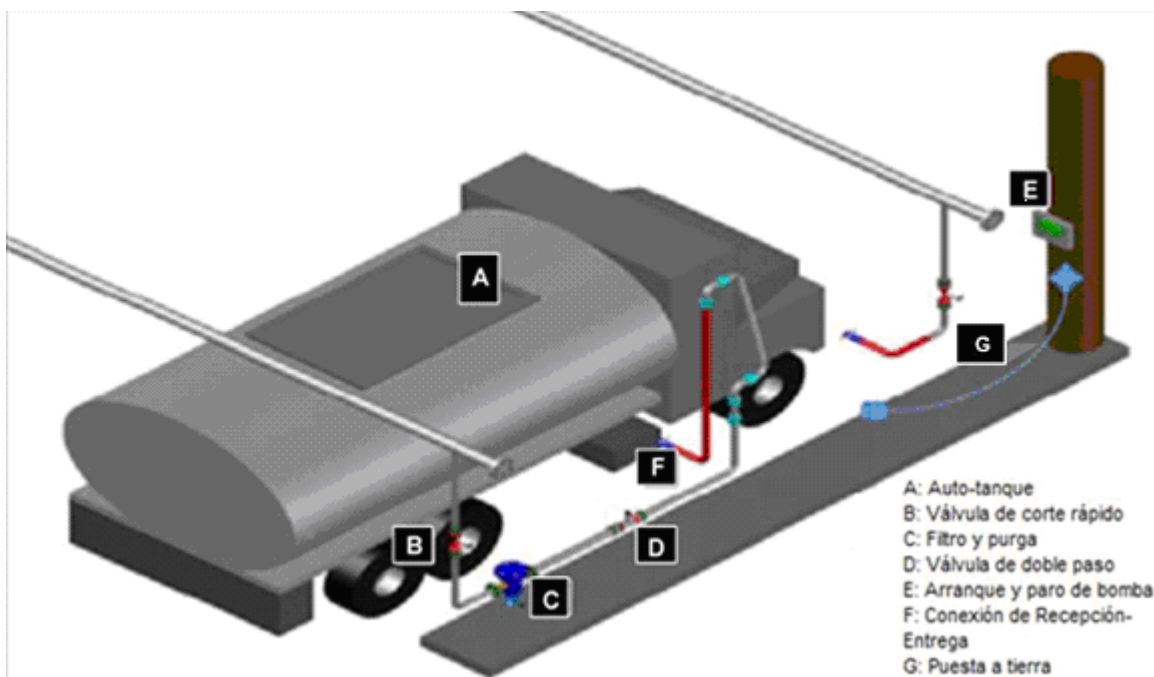
Figura 6. Sistema de Recepción y Entrega de Auto-tanques
