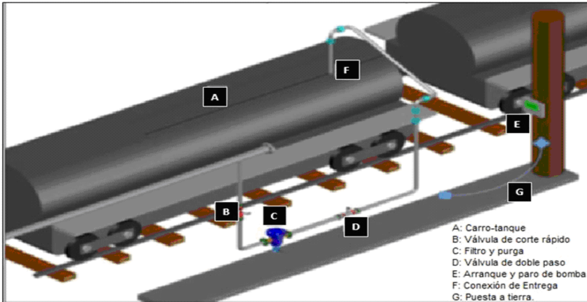
Figura 7. Sistema de Recepción de Carro-tanque
