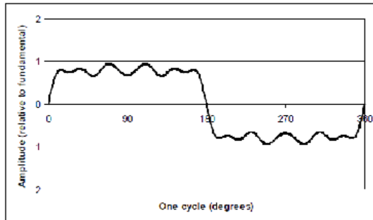
Figura 1. Amplitud de corriente para la forma de onda cuadriforme (en idioma inglés).
