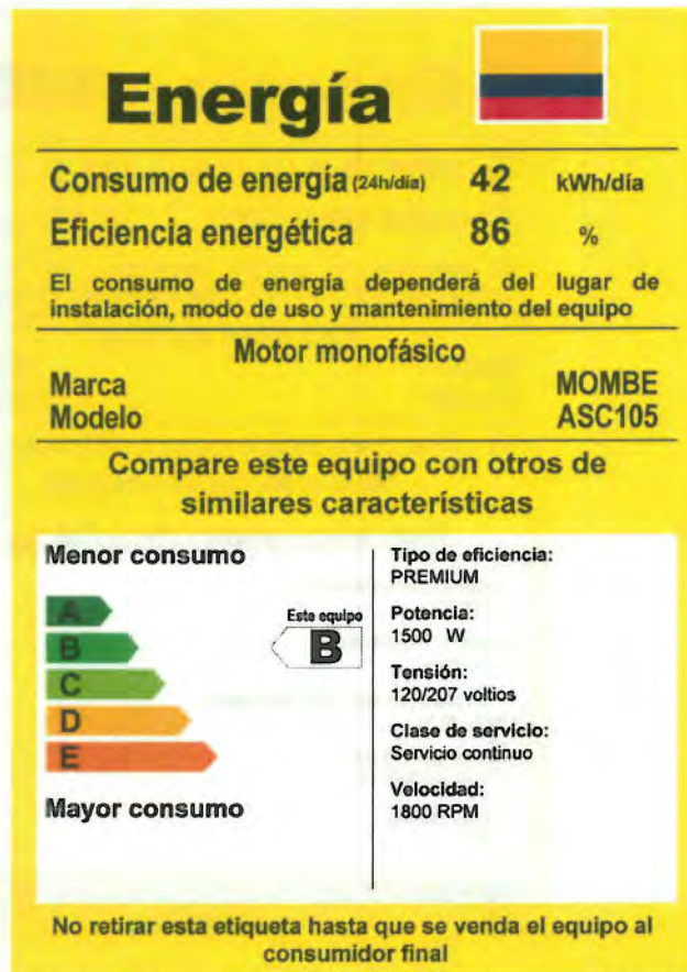
Figura 11.7. Ejemplo de etiqueta para Motores Monofásicos.
