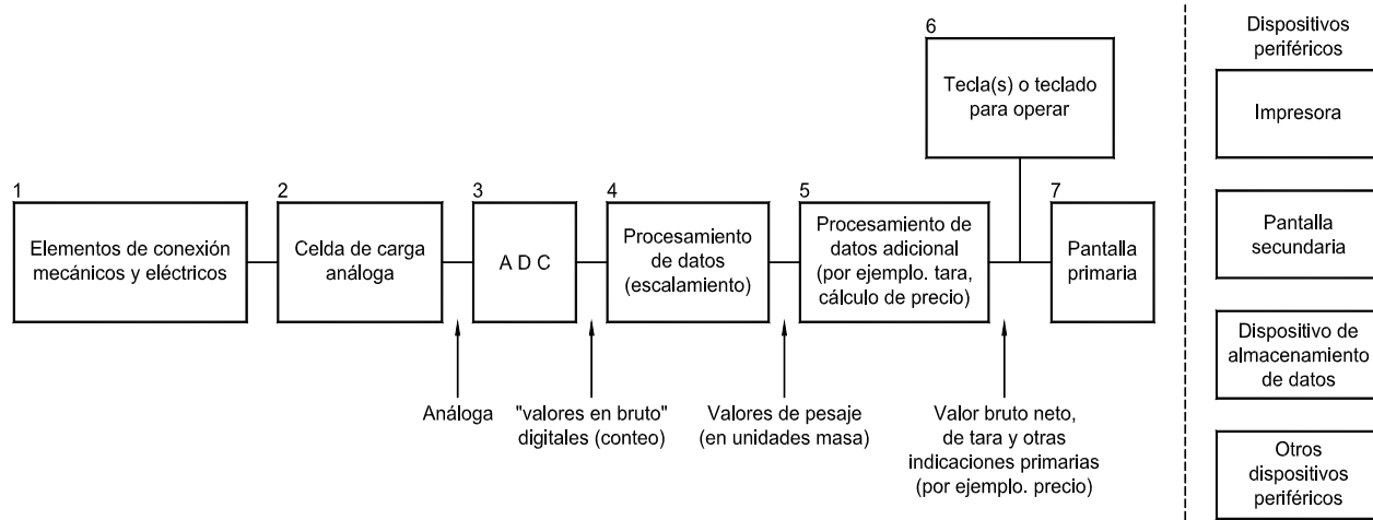
Figura 1 Definición de módulos típicos de acuerdo con T.2.2 y 3.10.2 (son posibles otras combinaciones)
