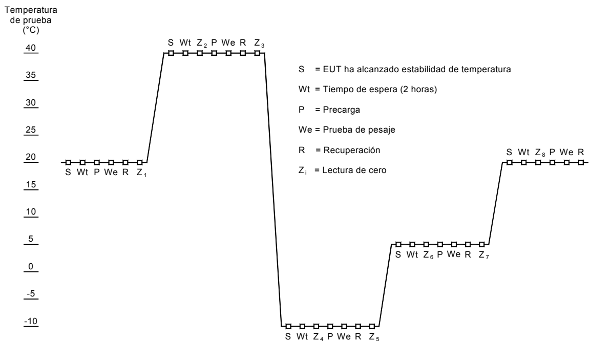
Figura 11. Secuencia de ensayo propuesta para el ensayo A.5.3.1 combinado con A.5.3.2 (ensayo de temperatura cuando los límites de temperatura son + 40 °C / - 10 °C)
