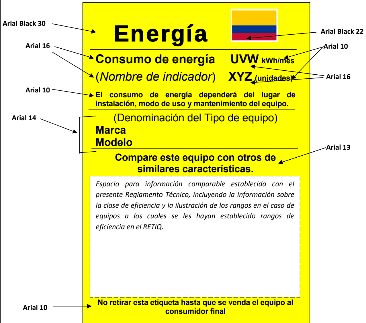
Figura 6.3.3. Ejemplo de dimensiones, distribución y tipos de letra a usar de una etiqueta normalizada (tamaño A6).
