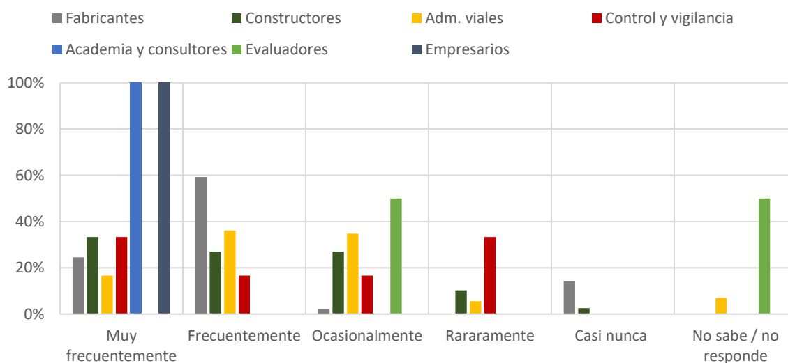
Ilustración 37. Influencia de los niveles de contención de sistemas de contención vehicular en afectaciones a los usuarios de las vías.
