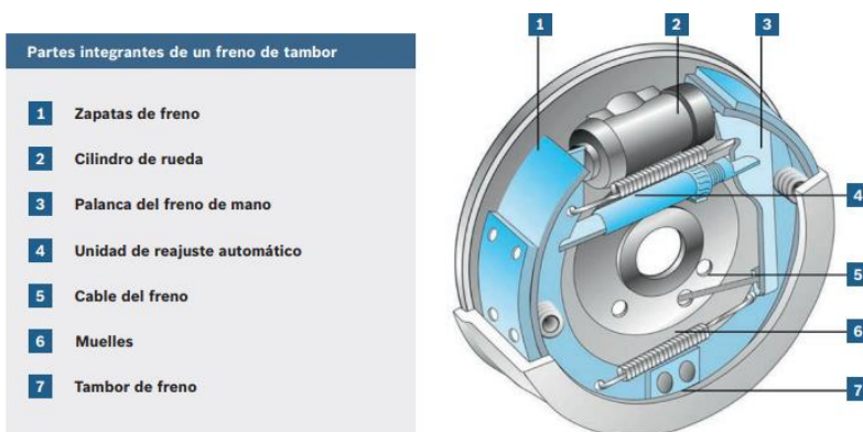
Ilustración 6 Frenos de Tambor, Luis Alvarado, Ford Motor Crafft, 2013.
