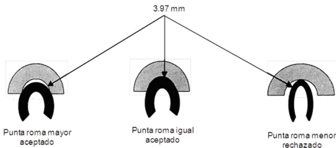
Figura 5 - Lectura de radio de punta roma
