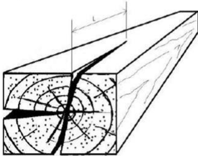
Figura 12. Pudrición.
