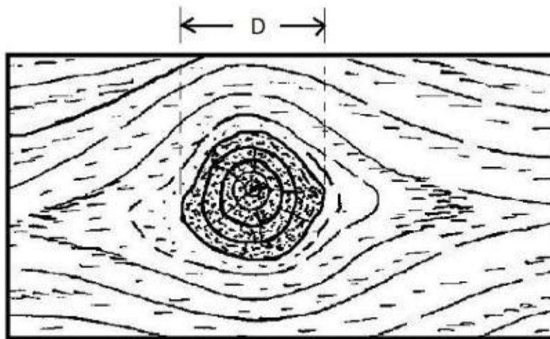
Figura 2. Nudo vivo
