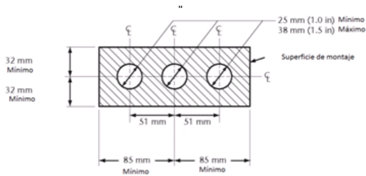
b) Griferías centrales normales de 100 mm
