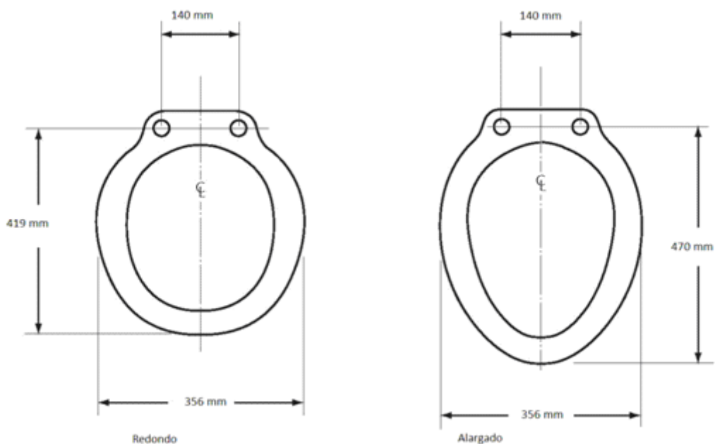
Figura 5.- Perfiles de tazas de inodoros
