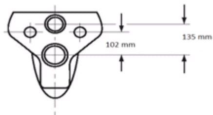
(b) inodoro de colgar con taza no sifónica y orificio de salida trasero.
