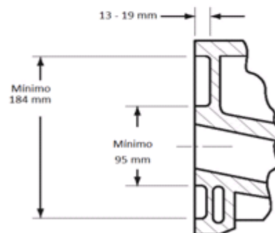
(d) Taza de inodoro para instalar en el piso con orificio de salida trasero
