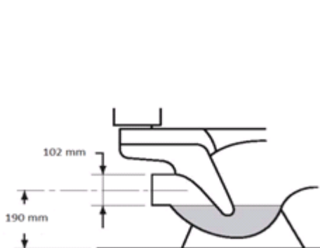
(c) Taza de inodoro para instalar en el piso con orificio de salida de espiga trasera.
