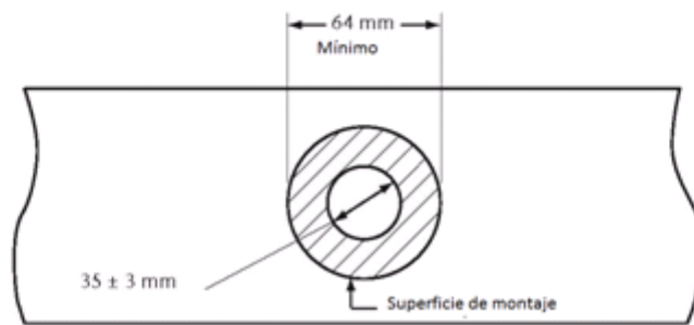
c) Grifería de montaje sencillo
