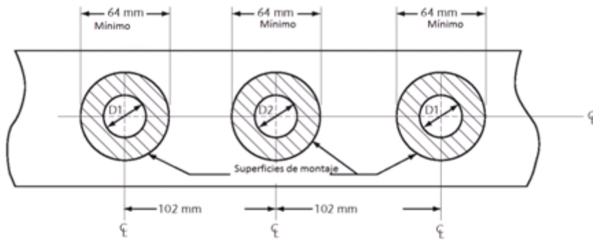
a) Griferías de combinación normales de 200 mm
